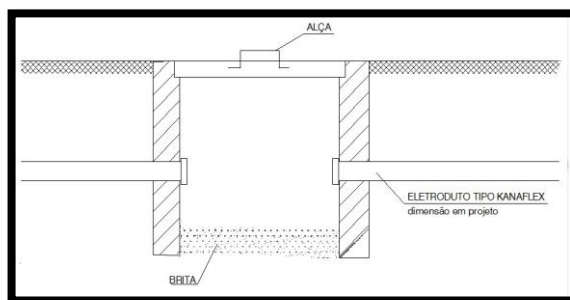
Figura 21 – Caixa de Passagem no piso
