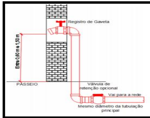
Figura 18 - Hidrante Recalque na fachada ou muro de divisa
