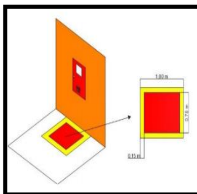
Figura 15 – Hidrante de Parede
